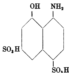
Aminonaphtoldisulfosäure K.
